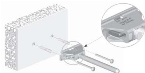
pritrnitev na betonsko steno
