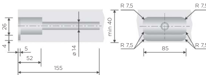
shema vrtanja
