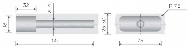
shema vrtanja za police debeline 25-30 mm
