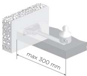
obremenitev + teža police = max 15 kg
