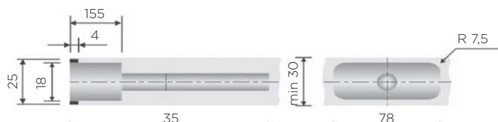
shema vrtanja za police debeline nad 30 mm
